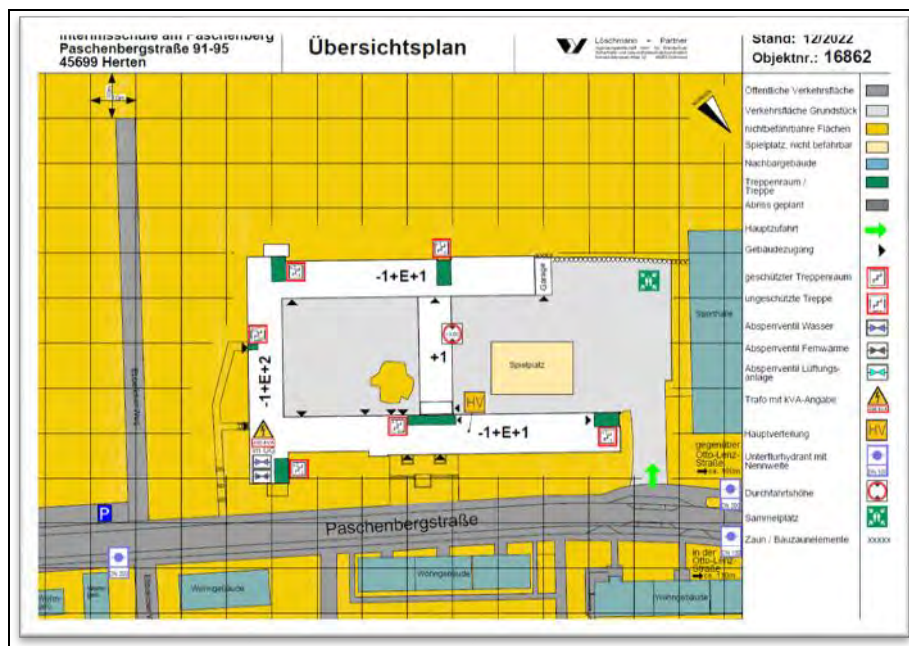
Bsp.:FW-Übersichtsplan „Interimsschule am Paschenberg“
