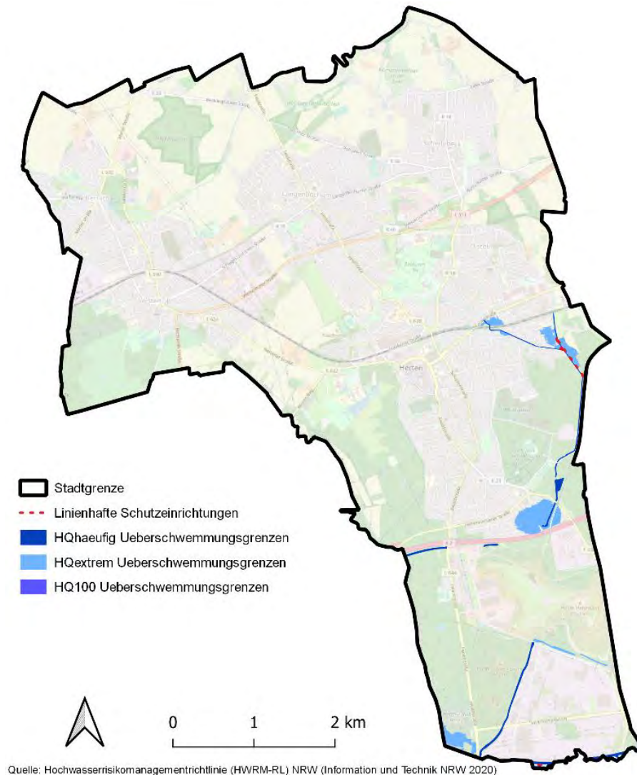
Abbildung 3-10: Hochwasserrisiko und Schutzmaßnahmen im Stadtgebiet Herten (Eigene Darstellung, Datengrundlage OpenGeodata NRW 2020)
